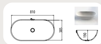
TB 0810 Aussenmaß: 840,5 x 432,2 mm
