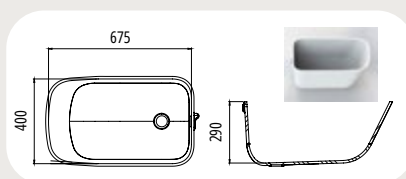
TB 0675 Aussenmaß: 724,3 x 423,8 mm
