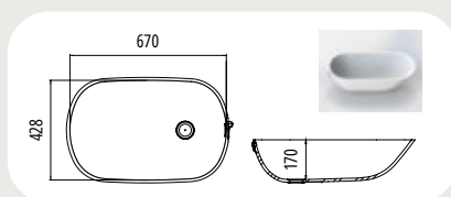
TB 0670 Aussenmaß: 713 x 453 mm
