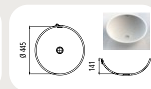
TR 0445 Aussenmaß: Ø 484 mm
