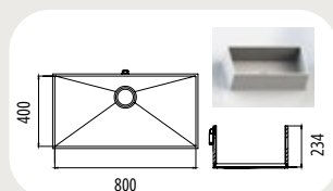
DTK 0800 Aussenmaß: 824 x 447 mm
