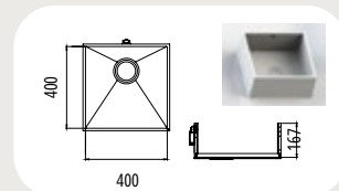
DTK 0400 Aussenmaß: 447 x 424 mm
