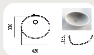
TE 0420 Aussenmaß: 444 x 380 mm
