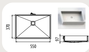
TP 0550 Aussenmaß: 574 x 422 mm
