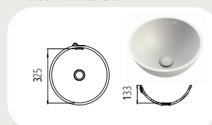
TR 0325 Aussenmaß: Ø 364
