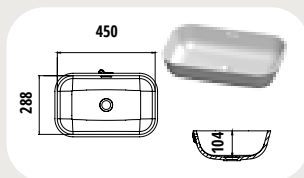
BS 288.450* NEU Aussenmaß: 312x474 mm
