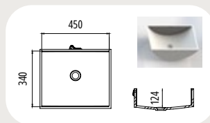
TL 0450-340* Aussenmaß: 484 x 404 mm
