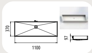
TP 1100 Aussenmaß: 1124 x 422 mm
