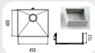
DTK 0450 Aussenmaß: 474 x 447 mm
