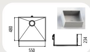
DTK 0550 Aussenmaß: 574 x 527 mm
