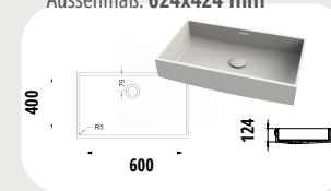
WDT 400.60* NEU Aussenmaß: 624x424 mm
